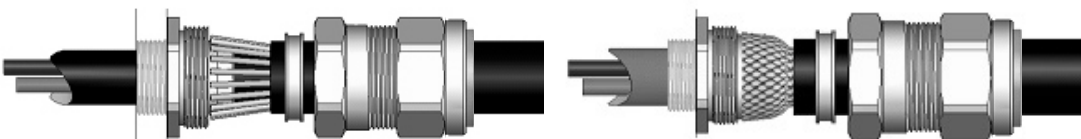
Армирование многожильным проводом
