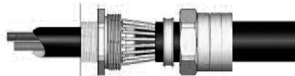
SWA Армирование многожильным проводом
